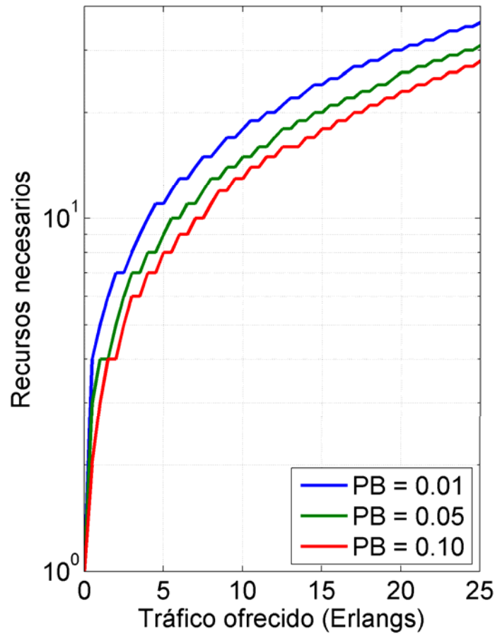
Servidores necesarios para un tráfico ofrecido dado
