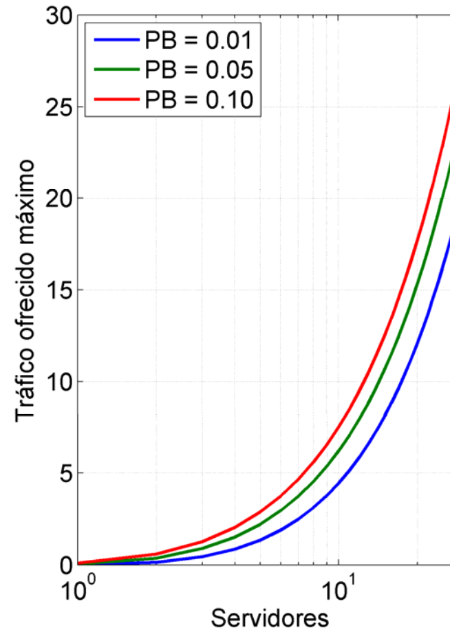
Tráfico máximo para un número de servidores dado
